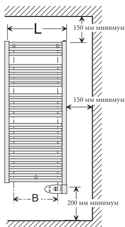
Вид спереди
