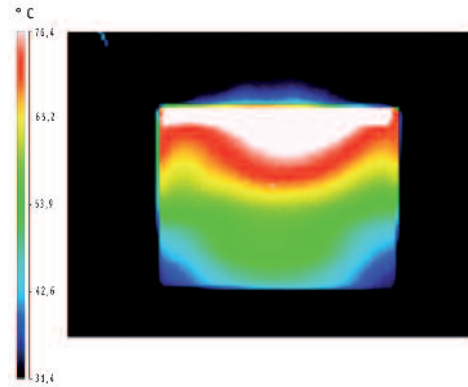
Равномерное распространение тепла конвекторов
